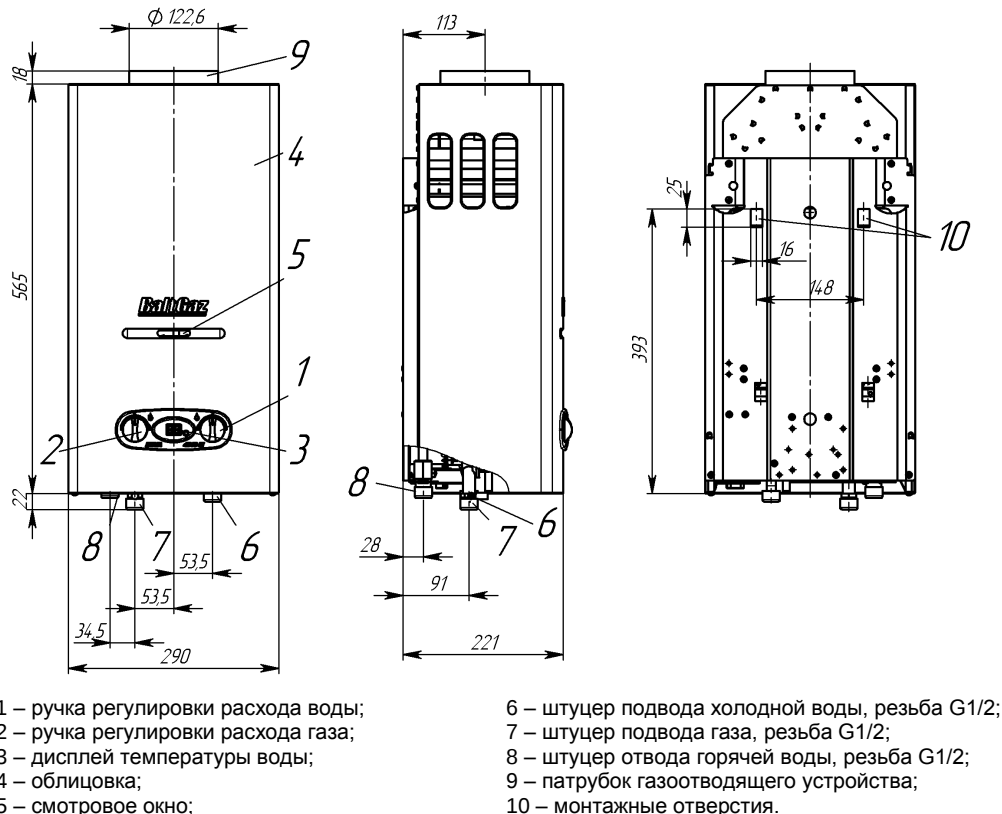
Рис. 1. Габаритные и присоединительные размеры аппарата
