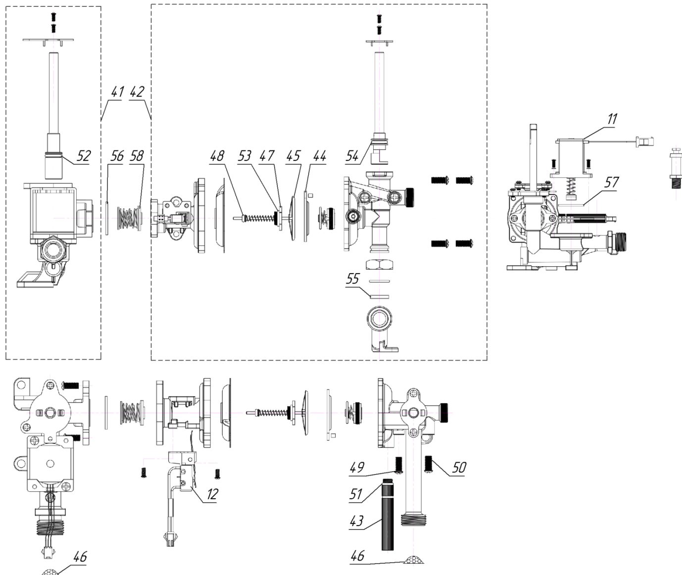
Рис. 11. Составные части узла водогазового 010623B806
