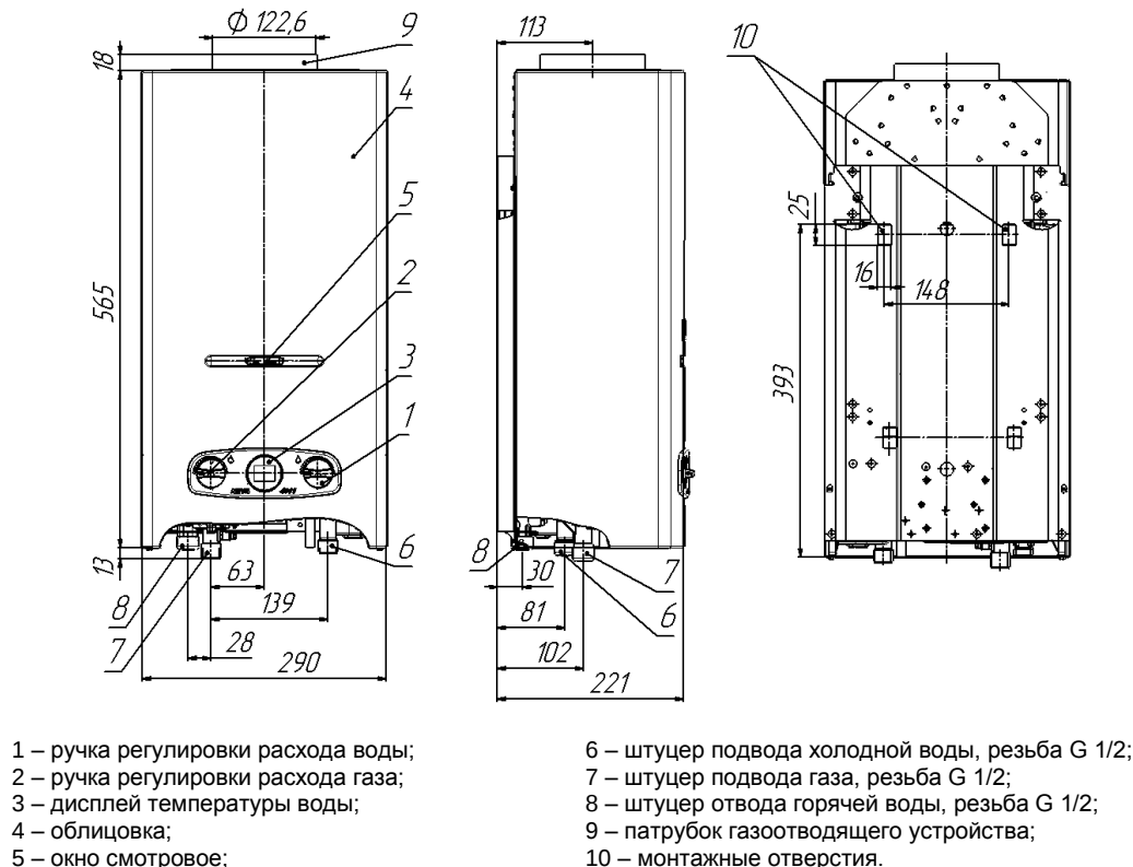
Рисунок 1. Габаритные и присоединительные размеры аппарата
