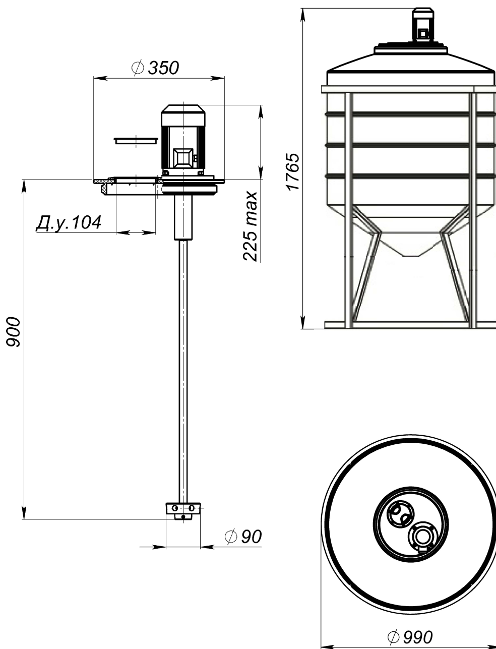
Габаритные размеры емкости ФМ 500 с установленной мешалкой
