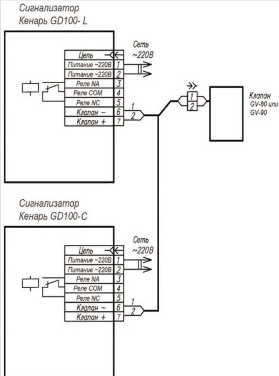
Схема соединения приборов
