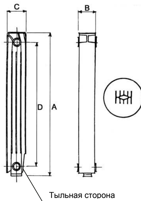
Рис. 1.1. Общий вид (а) и габаритные размеры (б) алюминиевого радиатора MUX
