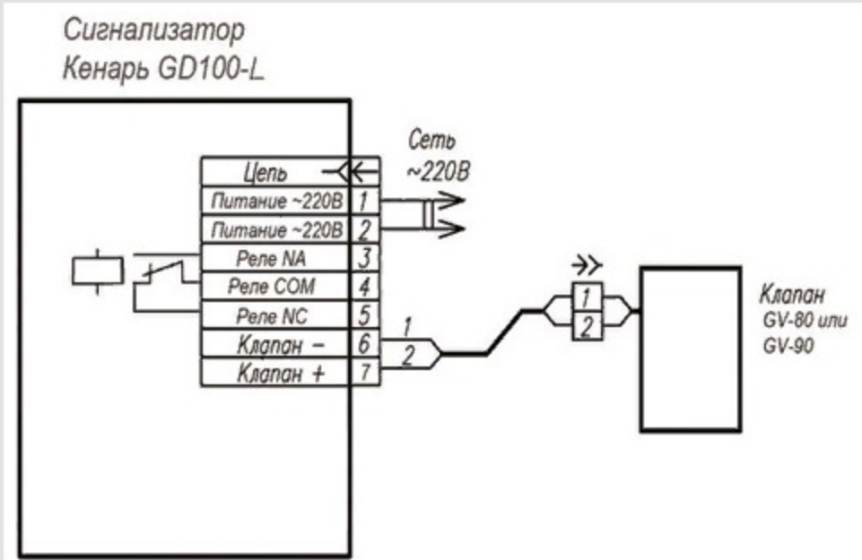
Схема соединения приборов
