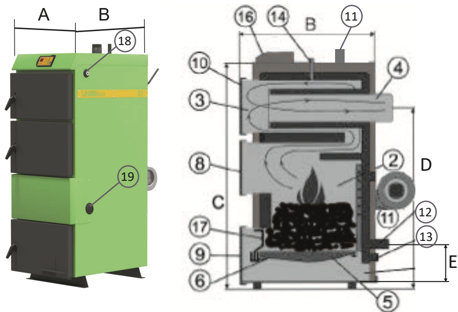
Рис. 1 котел «LavoGo XL»
