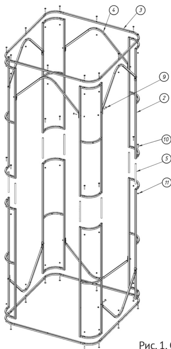
Рис. 1. Сборка каркаса.
